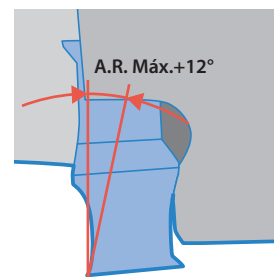
Borde Helicoidal con A.R. Max.+12°
