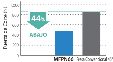
Borde Helicoidal con A.R. Max.+12°
